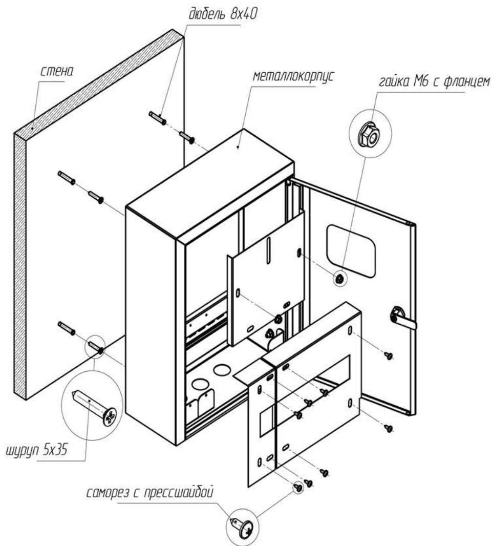
Рис. 1 - Схема монтажа
