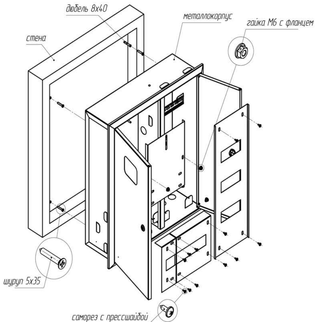
Рис. 1 - Схема монтажа
