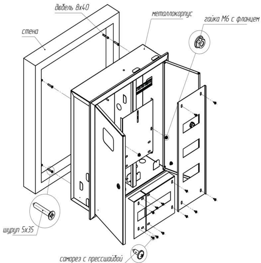
Рис. 1 - Схема монтажа
