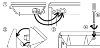
Рис. 3 Схема установки
