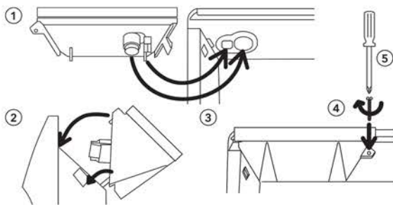
Рис. 3 Схема установки
