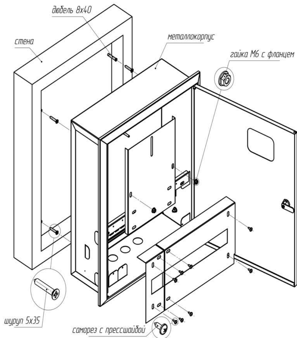
Рис. 1 - Схема монтажа
