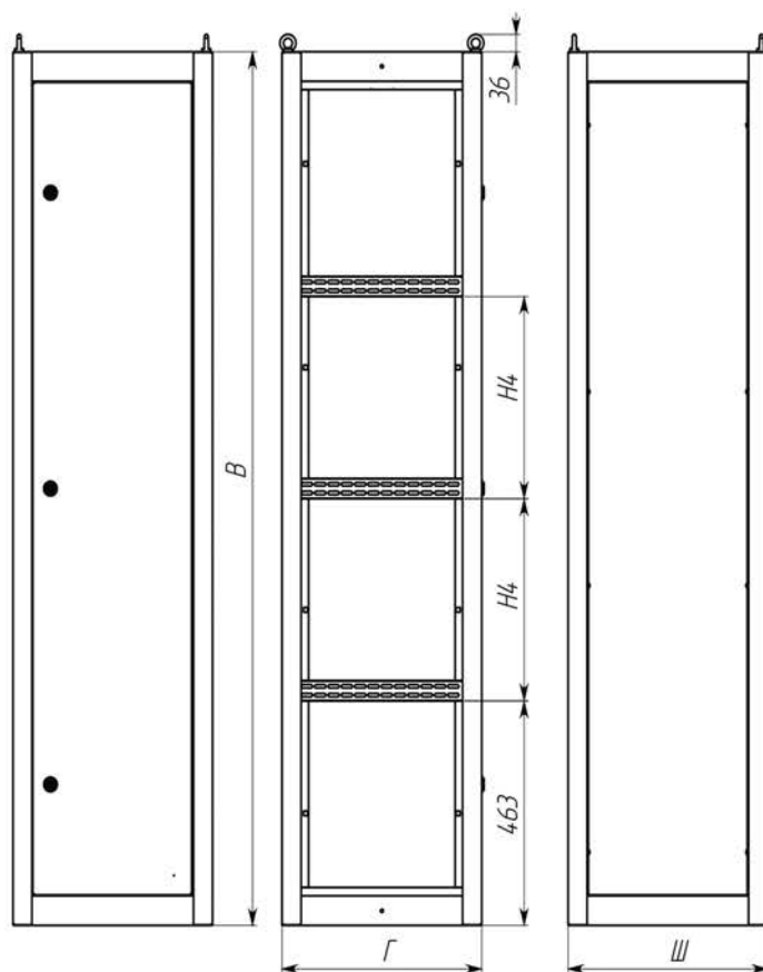
Рис.1 - Общий вид шкафов ВРУ-1 Unit S
