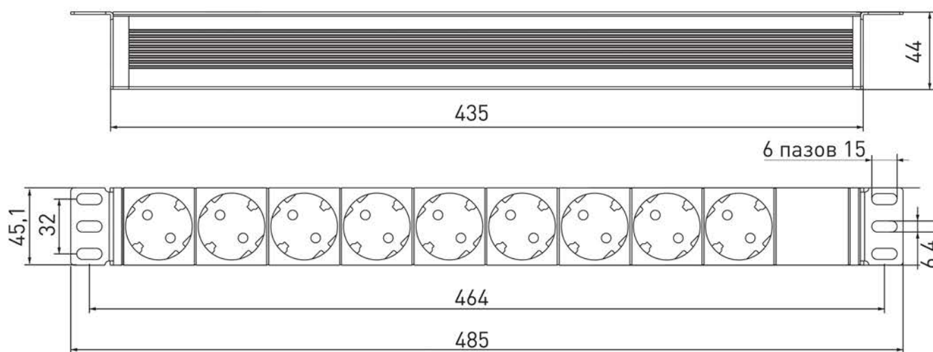
Рис. 1 Габаритные размеры блока розеток PDU TERACOM PRO (в мм)
