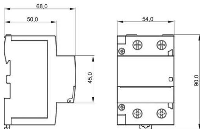
Рисунок 5 – Габаритные размеры контакторов 100 А, 2P / Figure 5 – Overall dimensions of 100 А, 2P contactors
