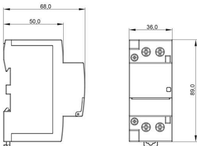
Рисунок 3 – Габаритные размеры контакторов от 40 А до 63 А, 2P / Figure 3 – Overall dimensions of contactors from 40 А to 63 А, 2P
