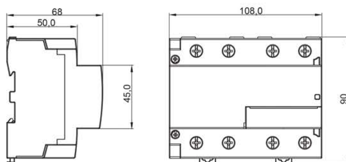
Рисунок 6 – Габаритные размеры контакторов 100 А, 4P / Figure 6 – Overall dimensions of 100 А, 4P contactors
