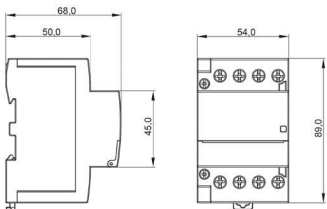
Рисунок 4 – Габаритные размеры контакторов от 40 А до 63 А / Figure 4 – Overall dimensions of contactors from 40 А to 63 А
