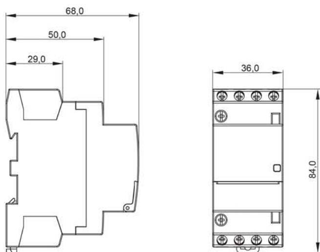
Рисунок 2 – Габаритные размеры контакторов до 25 А, 4P / Figure 2 – Overall dimensions of contactors up to 25 А, 4P
