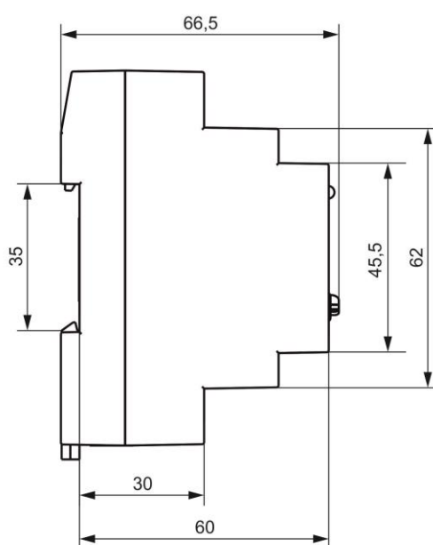
Рисунок 1 – Органы управления, габаритные и установочные размеры
