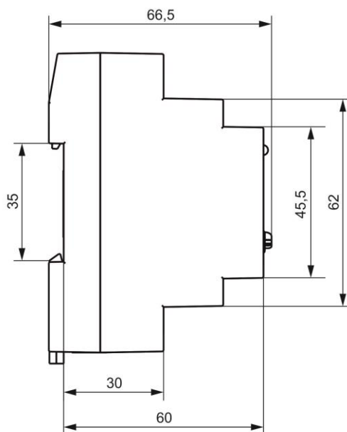
Рисунок 1 – Органы управления, габаритные и установочные размеры
