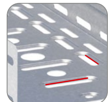
Продольная и поперечная подштамповка для увеличения площади охлаждения и придания дополнительной жесткости основанию лотка
