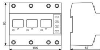
Рис.2. Габаритные размеры
