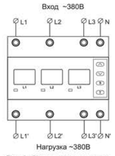
Рис.1. Схема подключения
