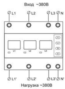
Рис.1. Схема подключения
