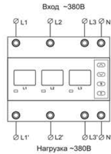
Рис.1. Схема подключения
