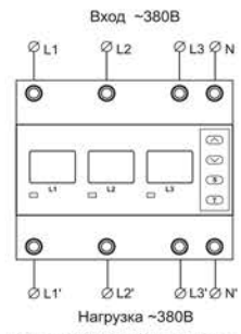
Рис.1. Схема подключения
