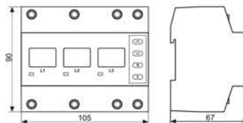
Рис.2. Габаритные размеры
