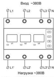
Рис.1. Схема подключения
