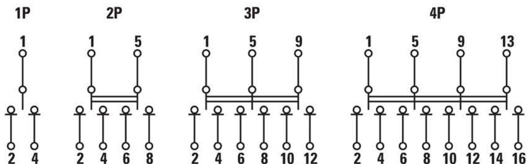
Рис. 2 - Принципиальная схема
