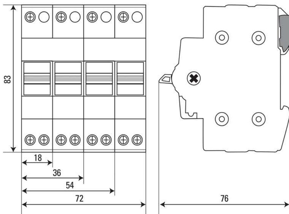
Рис.1 - Габаритные размеры
