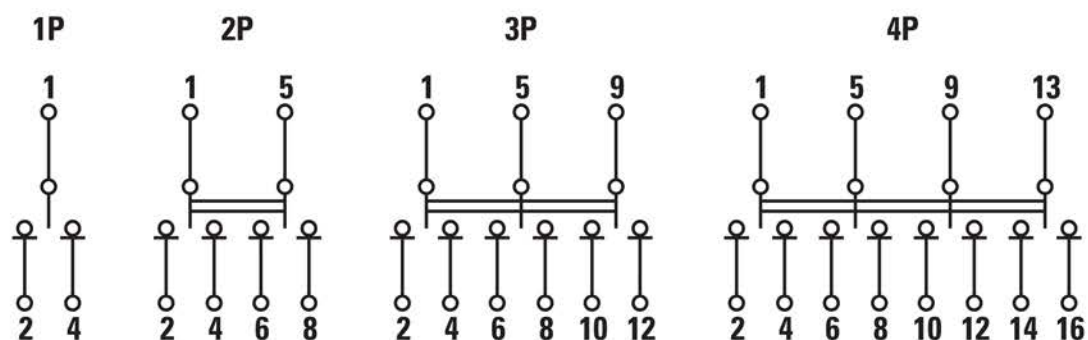
Рис. 2 - Принципиальная схема
