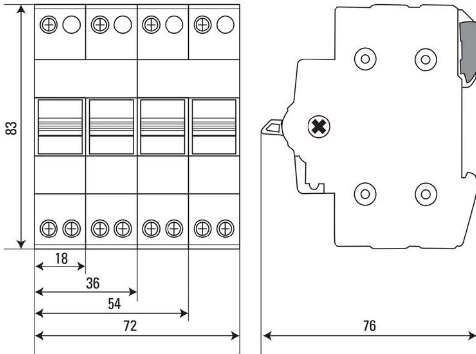
Рис.1 - Габаритные размеры
