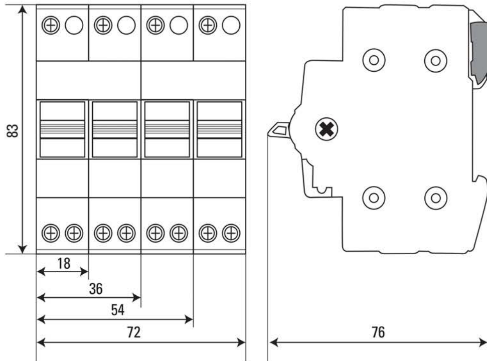
Рис.1 - Габаритные размеры
