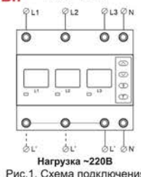
Рис.1. Схема подключения
