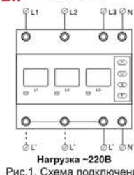
Рис.1. Схема подключения
