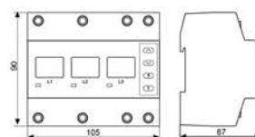
Рис.2 Габаритные размеры
