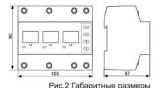
Рис.2 Габаритные размеры
