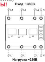
Рис.1. Схема подключения
