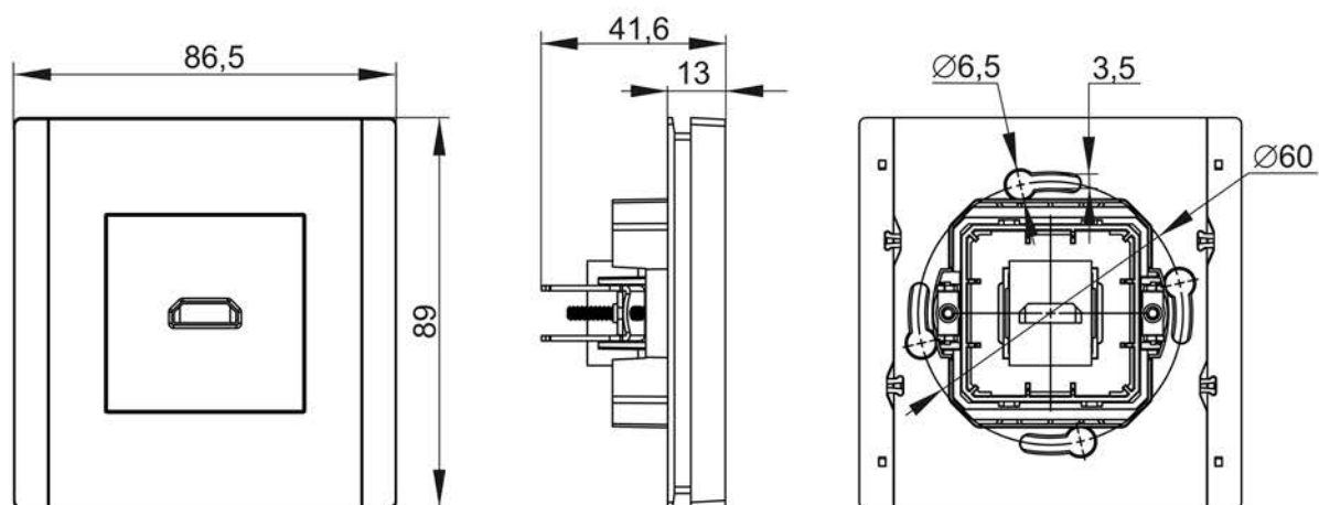
h) HDMI розетка / socket / priză / rozetka
