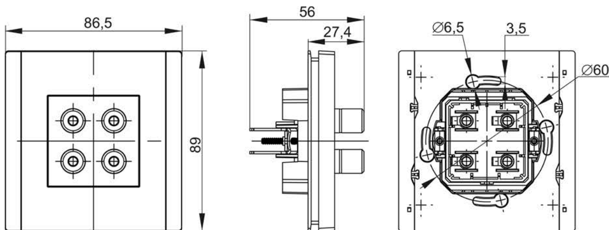
g) акустическая розетка / audio socket / акустикалық розетка / priza de acustică / акустикийн залгуур / akustik rozetka
