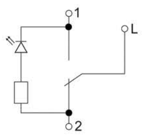
г) выключатель одноклавишный с индикацией / pass- through 1-gang switch with indication / индикациясы бар бір пернелі өтпелі ажыратқыш / intrerupator singură de trecere prin cu indicatie / нэг даралттай нэвт гаралтай led гэрэлтэй унтраалга / indikatsiyali o'tuvchi bitta klavishli o'chirgich
