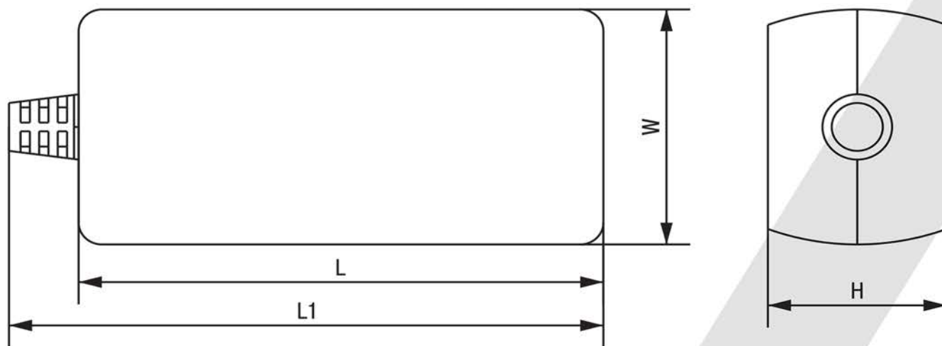
Рисунок 1 – Колодка удлинителя
