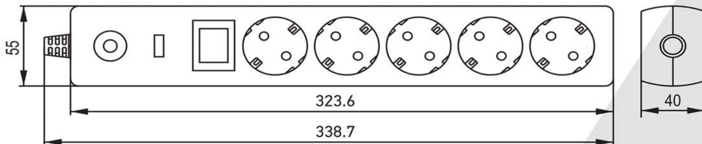
Рисунок 1 — Колодка фильтра на 5 мест
