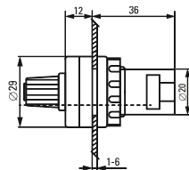
Потенциометр
