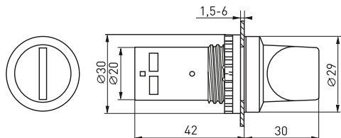
Переключатели SW2C-11X/2, SW2C-20X/3
