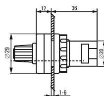
Потенциометр
