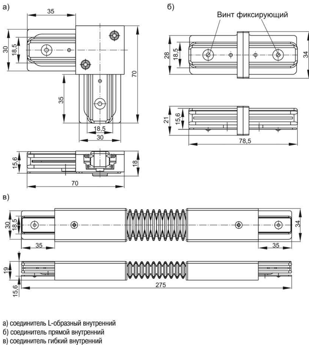
Рисунок 3 – Габаритные размеры соединителя
