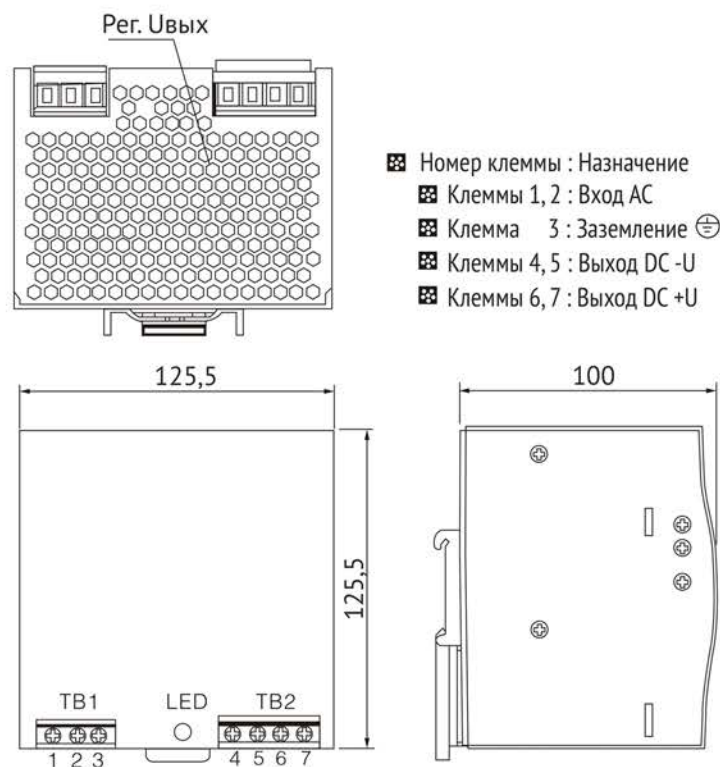
Рис.9 Габаритные размеры блоков питания DRP-240
