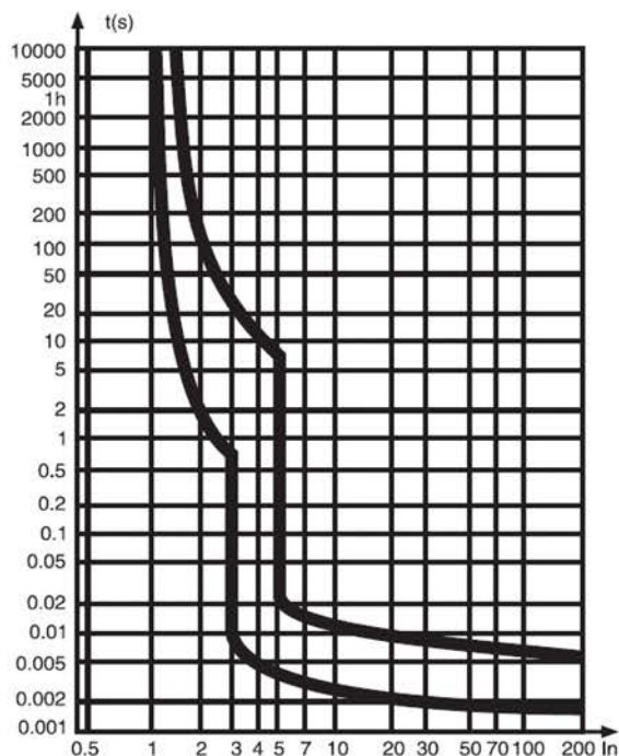
Рис. 1. Время-токовая характеристика В
