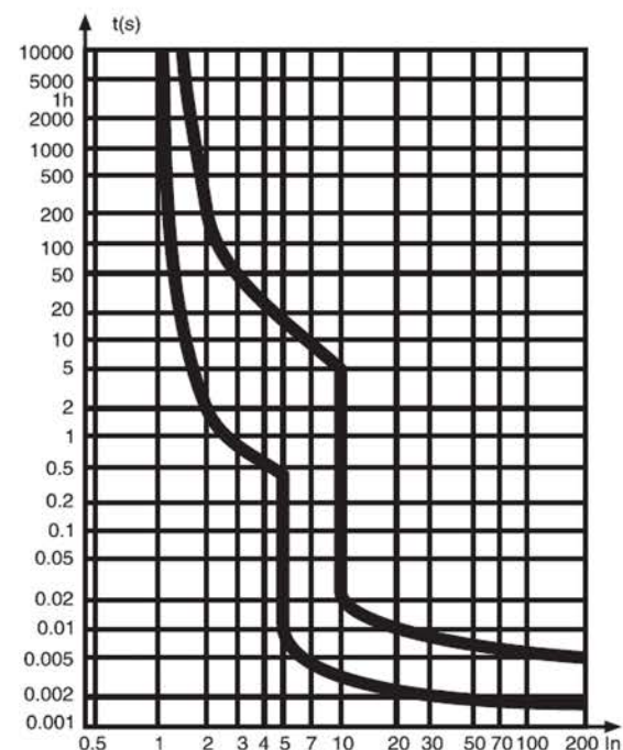
Рис. 2. Время-токовая характеристика С
