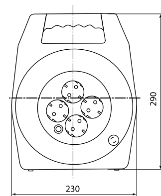
Удлинитель силовой в корпусе, 4 места
