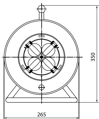
Удлинитель силовой с крышкой, 4 места
