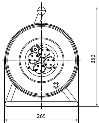
Удлинитель силовой, 40, 50 м, 4 места с проводом ПВС 3x1,0 мм 2 и ПВС 3x1,5 мм 2
