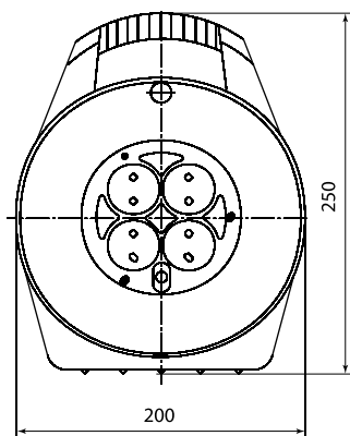
Удлинитель силовой в корпусе, 4 места
