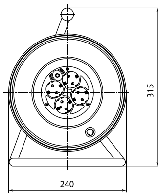
Удлинитель силовой, 30 м, 4 места с проводом ПВС 3x1,0 мм 2 и ПВС 3x1,5 мм 2
