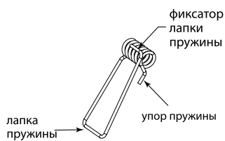
Конструкция пружины
