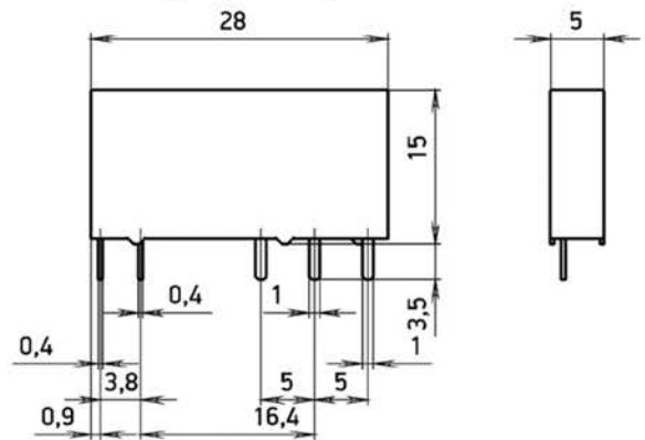
Рисунок Б.1 – Габаритные, установочные, присоединительные размеры реле OptiRel G RP34 с CO контактами
