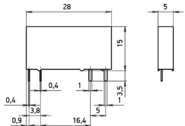
Рисунок Б.2 – Габаритные, установочные, присоединительные размеры реле OptiRel G RP34 с NO контактами
