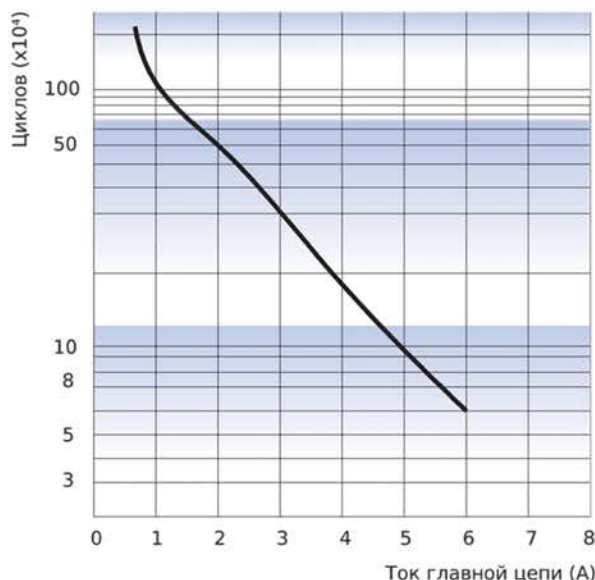
Рисунок Г.2 – Электрическая долговечность (AC) при номинальной нагрузке
