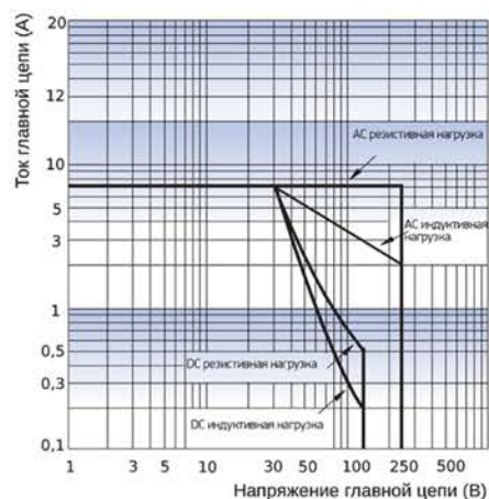
Рисунок Г.3 – Максимальная коммутируемая мощность для реле OptiRel G RP55-X2 и OptiRel G RP55-X3
