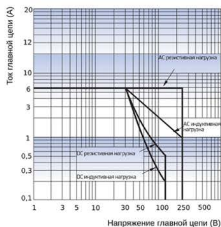
Рисунок Г.4 – Максимальная коммутируемая мощность для реле OptiRel G RP55-X4
