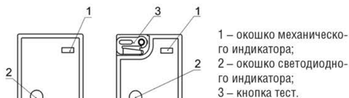
Рисунок Б.6 – Реле OptiRel G RP55 вид сверху
