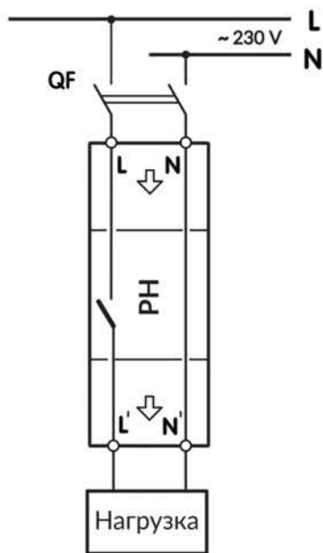
QF - двухполюсный автоматический выключатель
