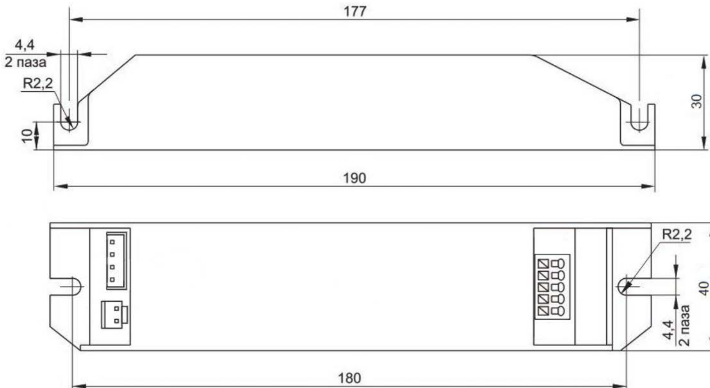
Рисунок 1 – Габаритные размеры БАП
