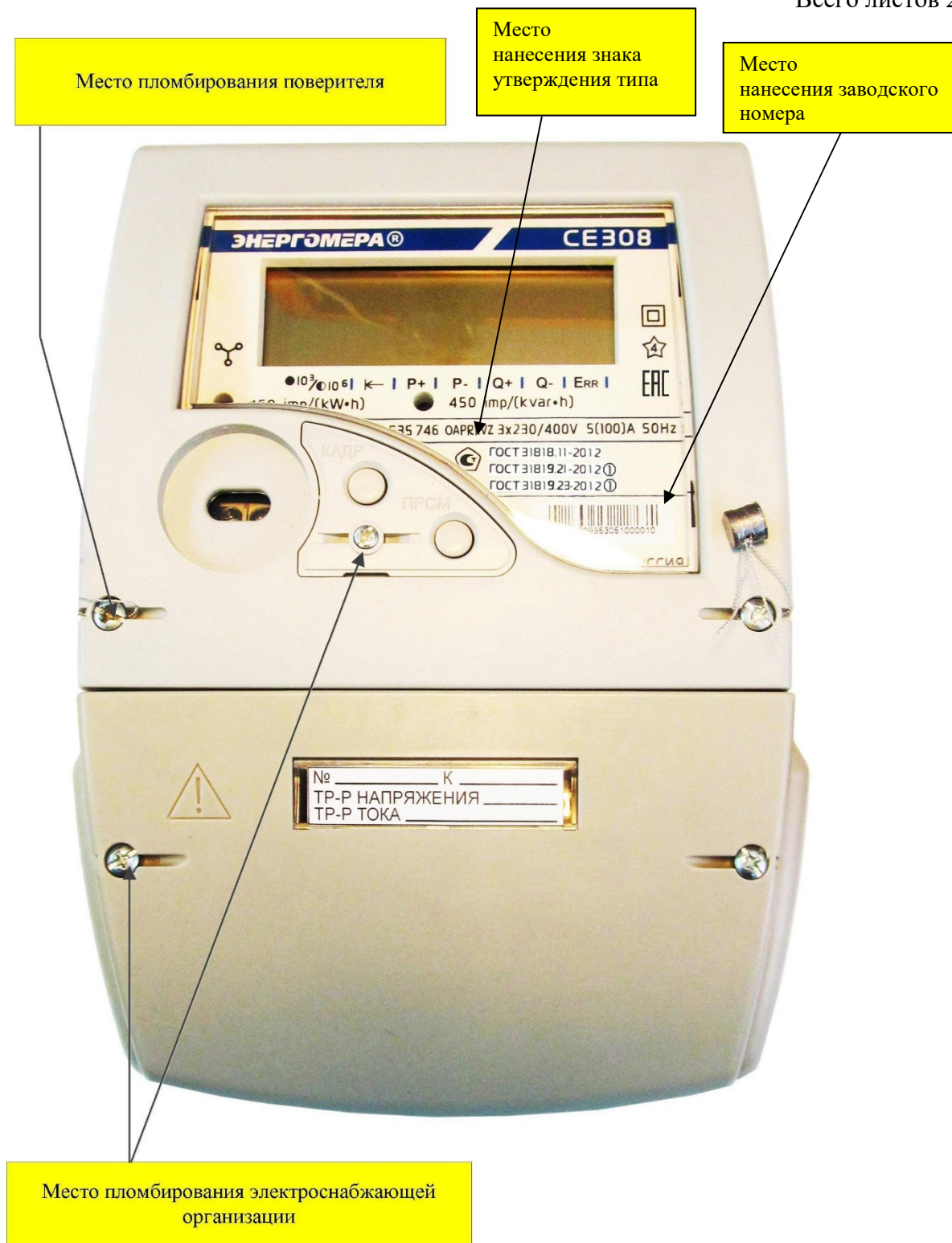
Рисунок 6 – Общий вид счетчика CE308 S35*
