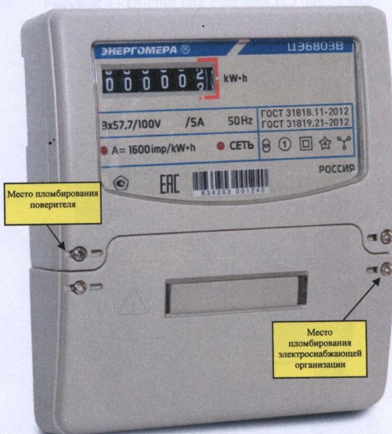
Рисунок 3 - Общий вид счетчика ЦЭ 6803В Р32
