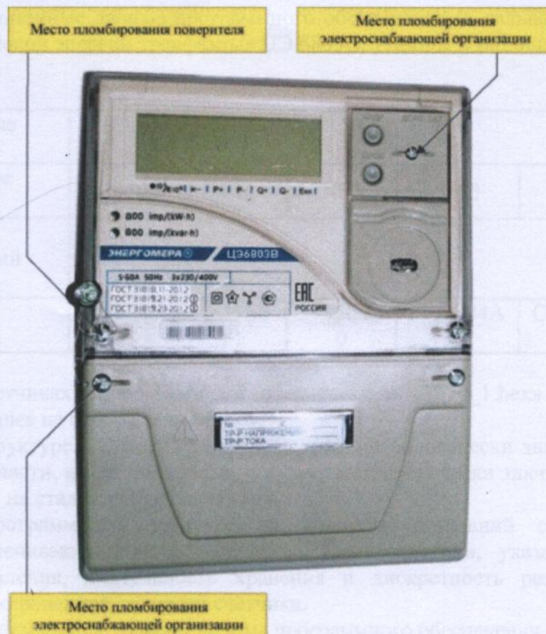
Рисунок 6 - Общий вид счетчика ЦЭ 6803В Ш31
