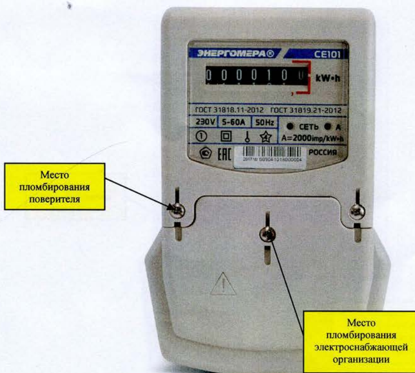
Рисунок 5 - Общий вид счетчика СЕ 101 S6
