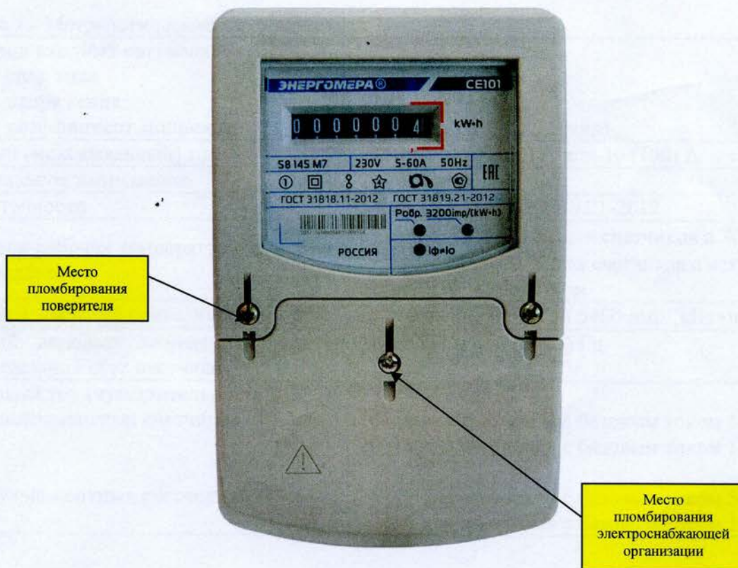
Рисунок 6 - Общий вид счетчика СЕ 101 S8
