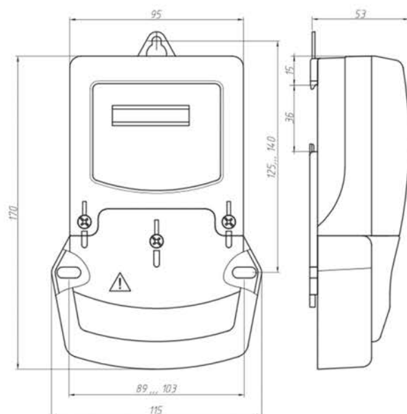
(тип корпуса S6)
