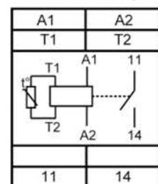
Рис. 2б 24DC
