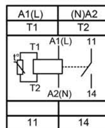
Рис. 2а AC230
