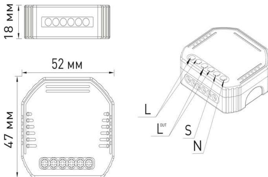
Рисунок 1. Общий вид и габаритные размеры диммера
