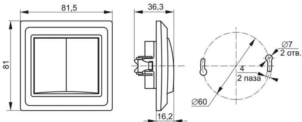
Рисунок 4 – Габаритные размеры выключателя BS10-2-0-ВБ
