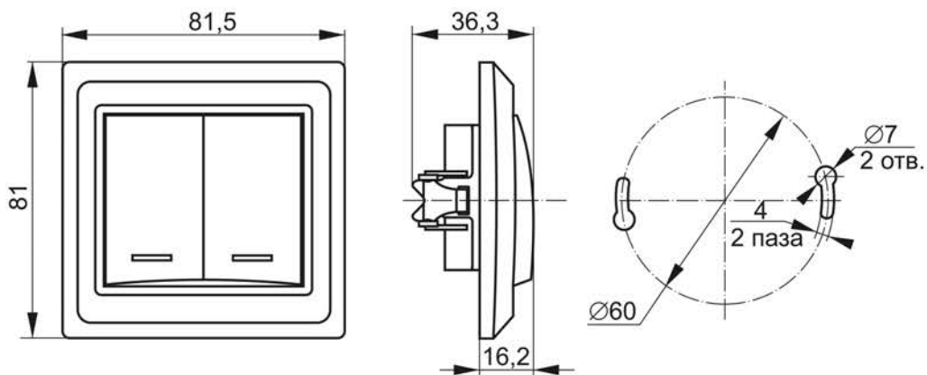
Рисунок 5 – Габаритные размеры выключателя BS10-2-1-ВБ
