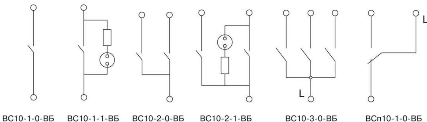
Рисунок 1 – Электрические схемы выключателей
