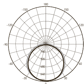
PWP-OS 1200 36w
