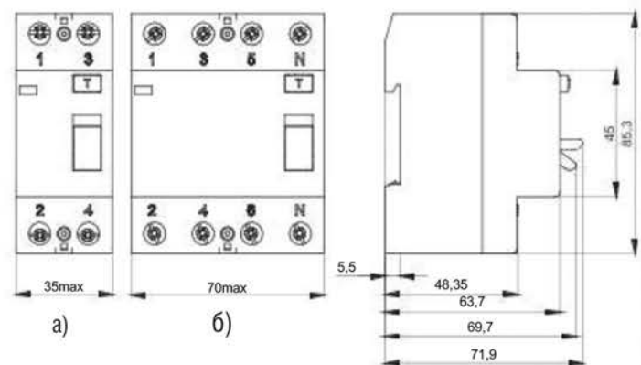
Рисунок Б.2 - Габаритные, установочные и присоединительные размеры ВДТ на номинальные токи 80-100А
