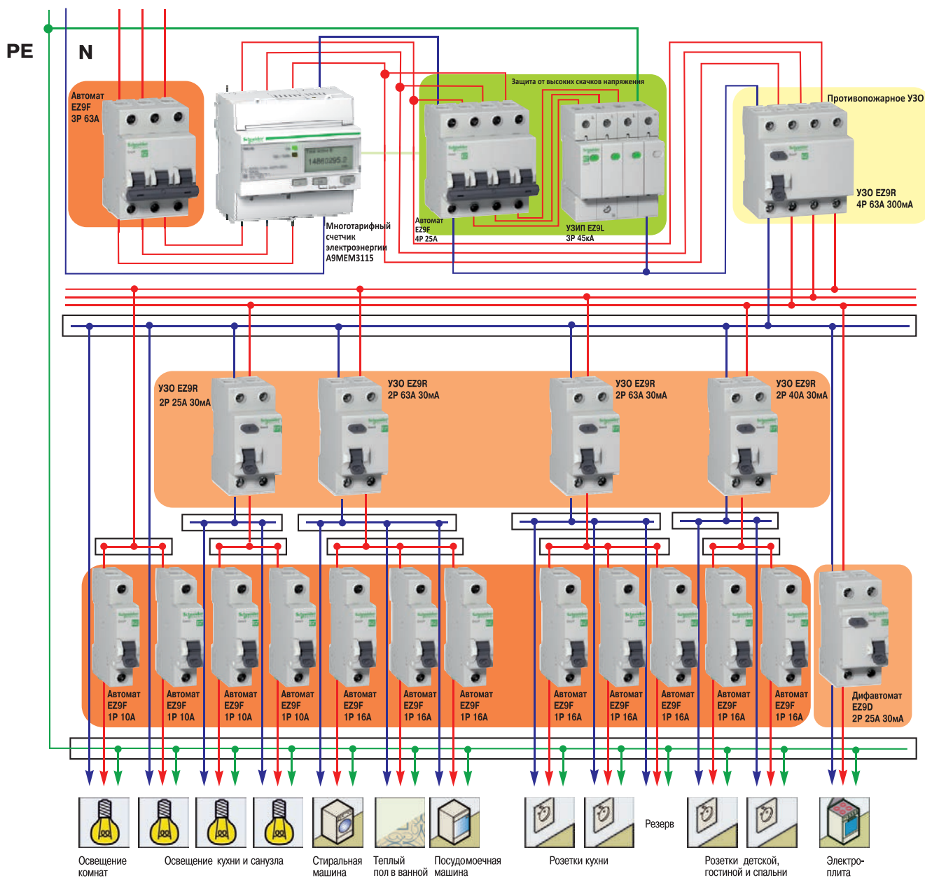
Пример схемы группового распределительного щита индивидуального здания (дома или дачи)
