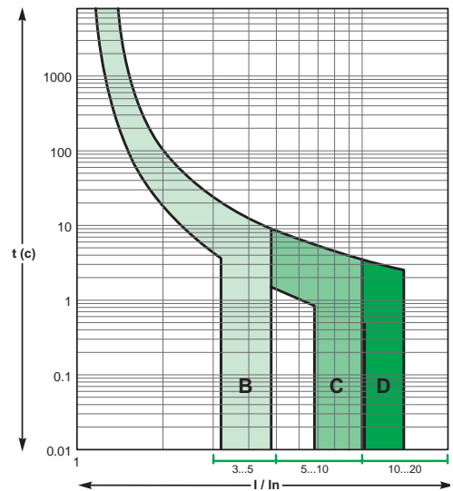
Кривые отключения
